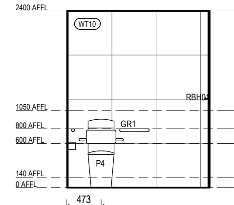
ACCESSIBLE WC 02 - 1
