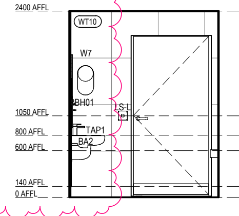
ACCESSIBLE WC 02 - 3
