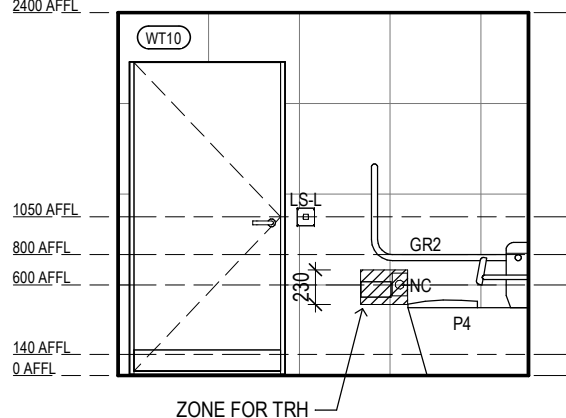
ACCESSIBLE WC 01 - 1
