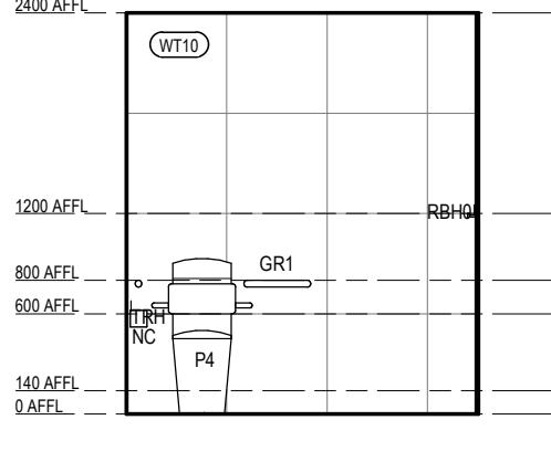
ACCESSIBLE WC 01 - 2
