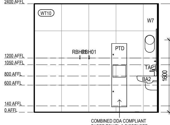
ACCESSIBLE WC 01 - 3
