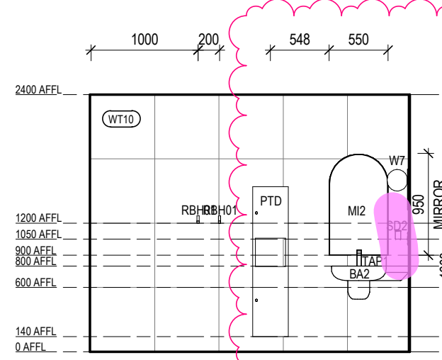
ACCESSIBLE WC 02 - 2
