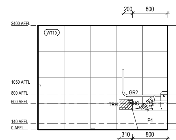
ACCESSIBLE WC 02 - 4
